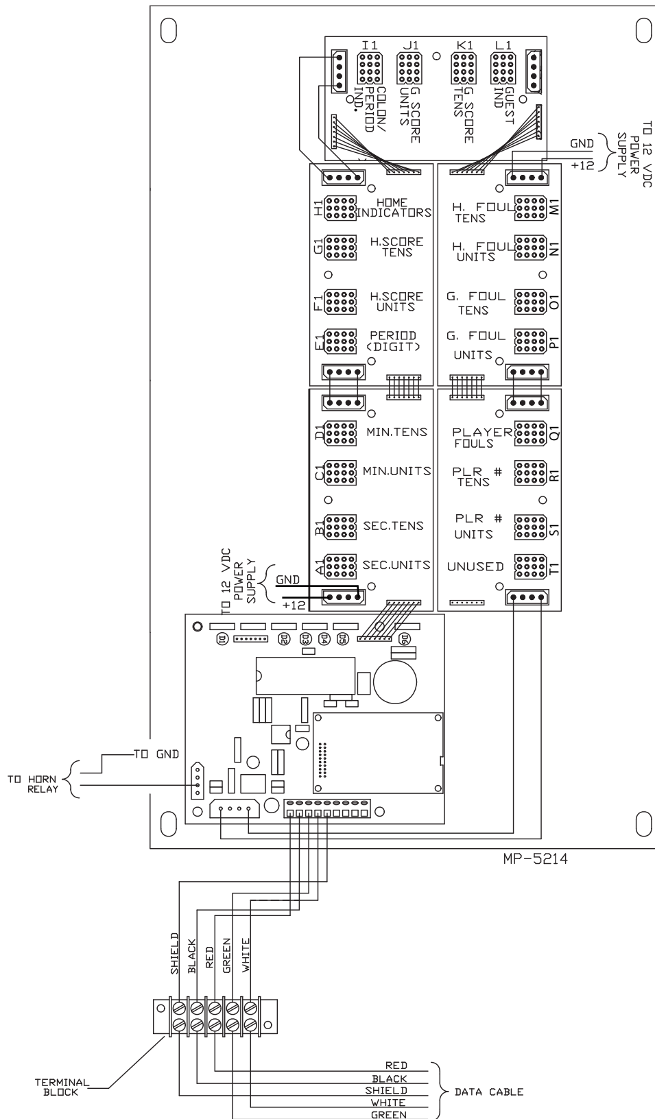
5214 Wiring Diagram
